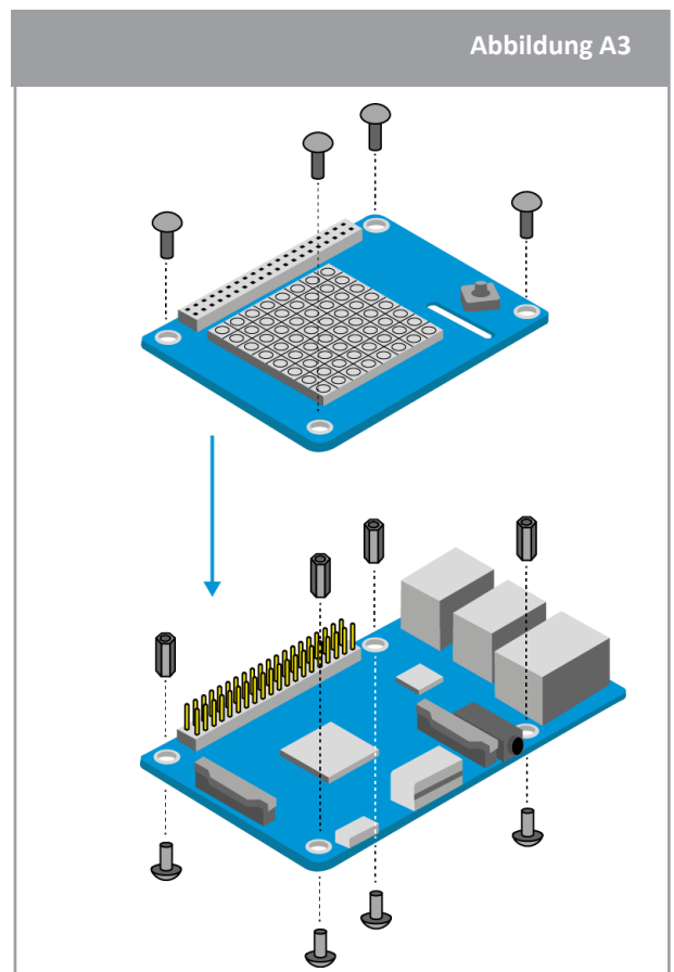
↑ Montage des Sense HAT am Raspberry Pi
