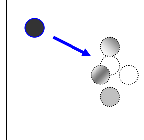
Die „Unschärferelation“
