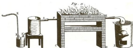
Abb. 31: Mit dieser Apparatur zerlegte Lavoisier Wasser über glühendem Eisen in Wasserstoff und Sauerstoff, wobei letzterer mit Eisen zu Eisenoxid reagierte („Thermolyse“)
