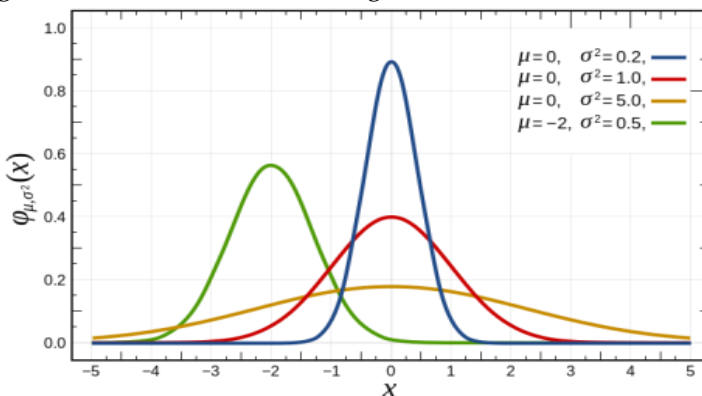
Abb. 49: Vier exemplarische Graphen der Dichtefunktion
