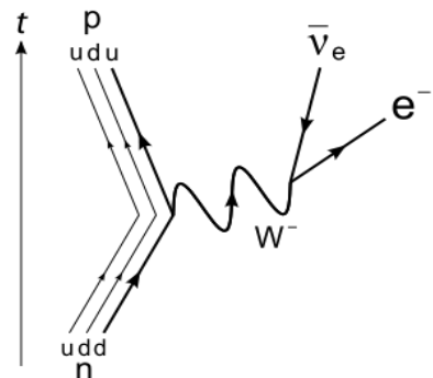
Abb. 91: Feynman-Diagramm vom Beta-Zerfall eines Neutrons n (aus den drei Quarks u , d und d ) in ein Proton p ( u -, d - und u -Quark), ein Elektron e^- und ein Elektron-Antineutrino \bar{\nu}_e über ein W -Boson
