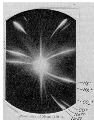
Abb. 39: Fotoplatte von 1913 mit den Isotopen von Neon ( 20 Ne und 22 Ne)
