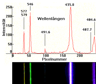
Abb. 65: Links Robert Wilhelm Bunsen (rechts) und Gustav Robert Kirchhoff , rechts das Spektrum einer Niederdruck-Quecksilberdampflampe, aufgenommen mit einem 256-Pixel-Zeilensensor bzw. mit einer Kamera
