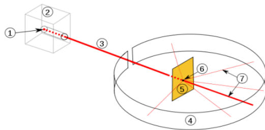
Abb. 80: Rutherfords Streuversuch 1911
