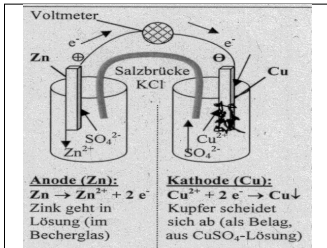
Abb. 13: Galvanisches Element aus Zink und Kupfer
