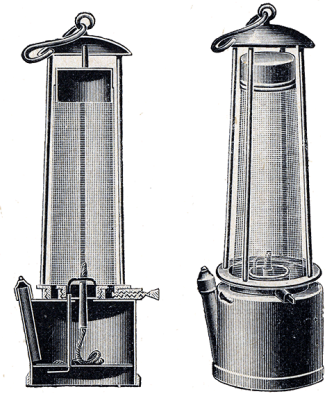
Fig. 192. Davysche Sicherheitslampe
