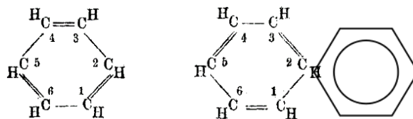
Abb. 61: Benzol C_6H_6 in der historische Formel von Kekulé , rechts daneben in der modernen Symbolschreibweise von Armit und Robinson .
