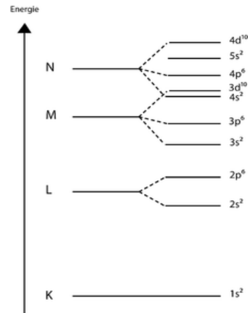
Abb. 84: Termschema, mögliche Energieniveaus von Elektronen im Atom
