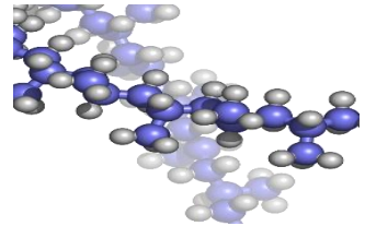
Abb. 97: Ausschnitt aus einem PP-Molekülmodell (Kugel-Stab-Modell)
