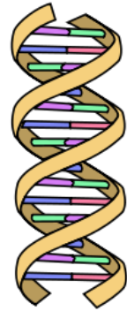
Abb. 101: Die Struktur des DNS-Moleküls – eine Doppelhelix
