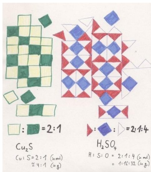
Abb. 32: Konstante Fliesenverhältnisse in bestimmten Fliesenmustern zur Veranschaulichung des Gesetzes der konstanten Proportionen, hier am Beispiel der Stoffmengen-Verhältnisse von Kupfer(I)-sulfid ( \text{Cu}_2\text{S} mit n(\text{Cu}) : n(\text{S}) = 2 : 1 ) und von Schwefelsäure ( \text{H}_2\text{SO}_4 mit n(\text{H}) : n(\text{S}) : n(\text{O}) = 2 : 1 : 4 ).
