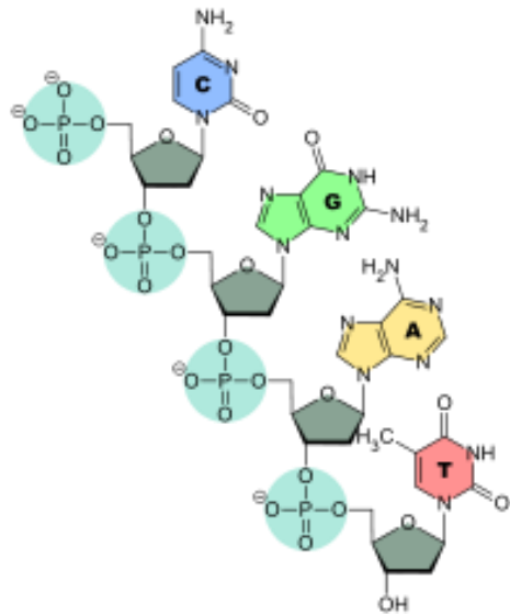
Abb. 76: Nukleinsäure-Bruchstück aus vier Ket tengliedern (hier: vier Nukleobasen A, C, G und T für Adenin, Cytosin, Guanin und Thymin, vier fünfeckige Zucker-Bausteine und vier Phosphat-Bindeglieder \text{PO}_4^{3-} )
