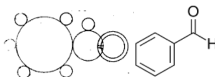
Abb. 38: Loschmidts „Constitutionsformel“ für Benzaldehyd C_6H_5-CHO (links), rechts die heutige Schreibweise.
