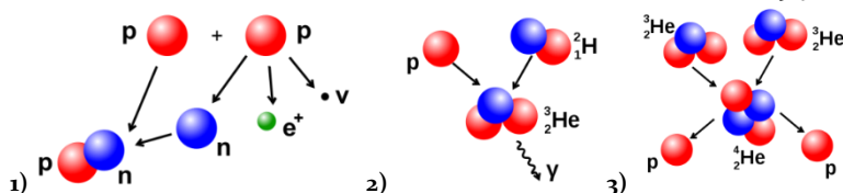
Abb. 94: Das „Wasserstoffbrennen“ (die Proton-Proton-Reaktion) – die Energiequelle der Sterne: Zwei Protonen ergeben einen Deuteriumkern, dieser bildet im zweiten Schritt mit einem weiteren Proton ein Helium-3-Nuklid, und zwei Helium-3-Nuklide ergeben einen stabilen Helium-4-Atomkern und zwei Protonen. Zusätzlich werden ein Positron e^+ und ein Neutrino \nu frei und harte Gammastrahlung (Photonen, ihr Symbol: \gamma ).
