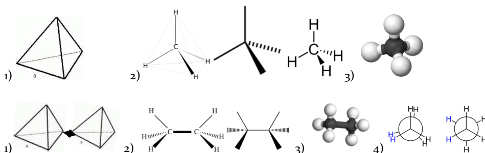
Abb. 54: Methan- und Ethanmoleküle im Tetraedermodell in verschiedenen Darstellungsweisen: Methan \text{CH}_4 (oben) und Ethan \text{H}_3\text{C}-\text{CH}_3 (unten) in: 1) Tetraedermodell 2) Keilstrichschreibweise 3) Kugel-Stab-Modell 4) Newman -Projektion
