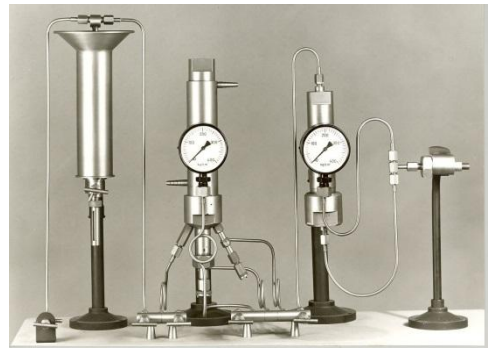
Abb. 98: Versuchsanordnung zur Herstellung von Ammoniakgas \text{NH}_3 aus den Elementen
