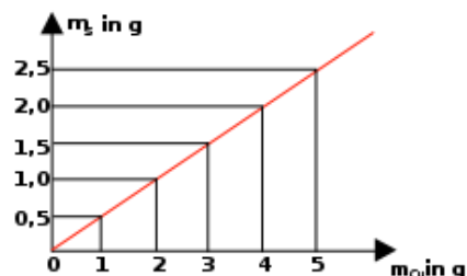
Abb. 2.14: Diagramm des Masseverhältnisses m(\text{Cu}) : m(\text{S}) = 2 : 1 im Kupfer(II)-sulfid (Abb. gemeinfrei)
