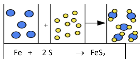
Abb. 1.21: Bildung von Pyrit \text{FeS}_2 aus Eisen- und Schwefelteilchen \text{Fe} + \text{S} im Masseverhältnis von: m(\text{Fe}) : m(\text{S}) = 7:8 (das entspricht einem Mengenverhältnis von n(\text{Fe}) : n(\text{S}) = 1:2 )
