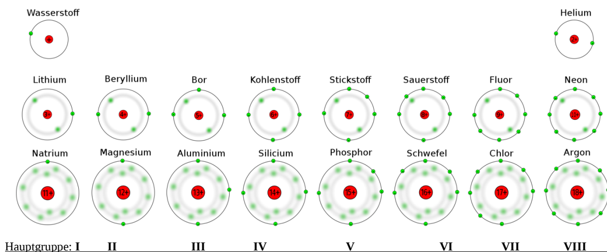
Abb. 3.5: Darstellung der Elemente Nr. 1-18 im Schalenmodell (Atommodell nach Bohr, Abb. gemeinfrei)
