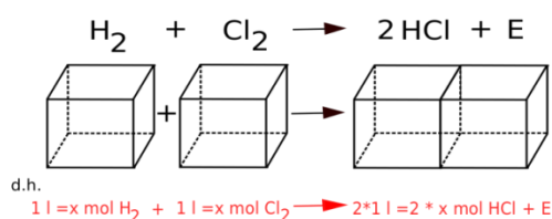
Abb. 1.22: Wasserstoffgas \text{H}_2 und Chlorgas \text{Cl}_2 reagieren zu Chlorwasserstoffgas \text{HCl} im Volumenverhältnis 1 : 1
