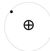
Abb. 3.3: Modell des H-Atoms: p + im Kern, e - in der Hülle (Eig. Abb.)
